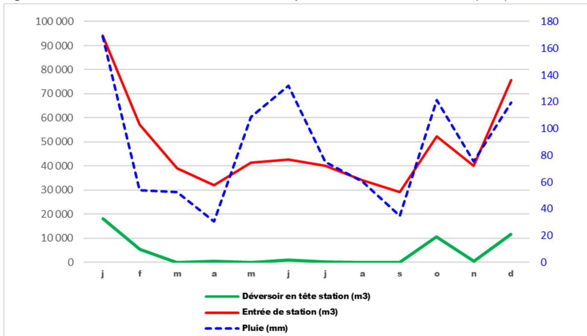
Figure 2 : Evolution mensuelle des volumes et de la pluviométrie en entrée de STEU (2021)
