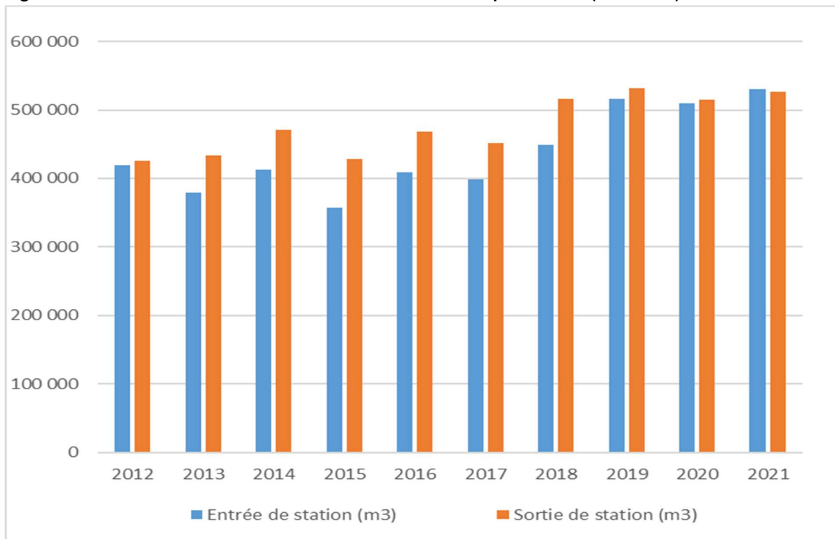
Figure 3 : Evolution annuelle des volumes en entrée et traités par la STEU (2012-2021)
